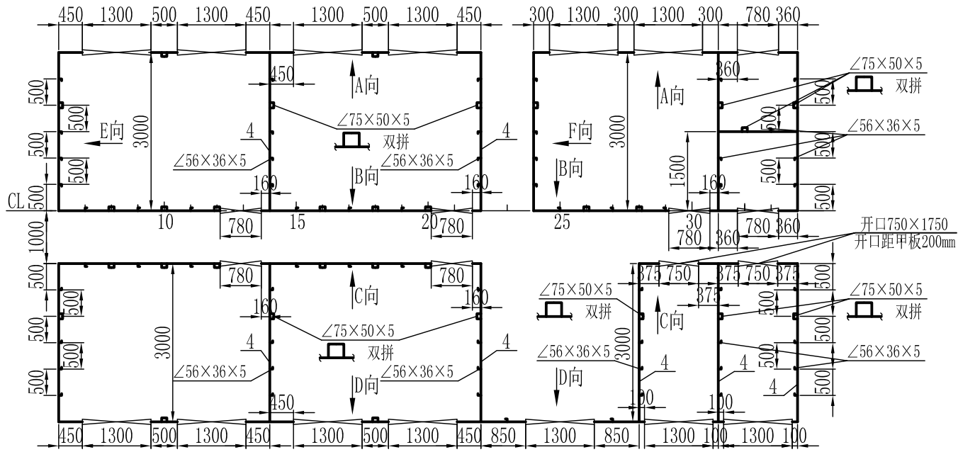
主甲板围壁平面图
