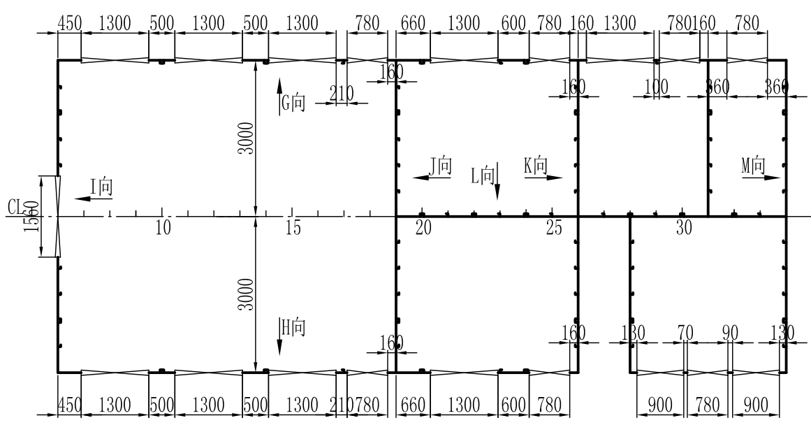
上甲板围壁平面图
