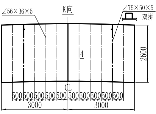
强横梁及甲板纵桁处 围壁扶强材连接形式
