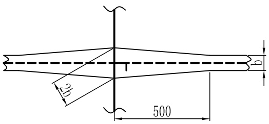
强横梁及甲板纵桁处 围壁扶强材连接形式
