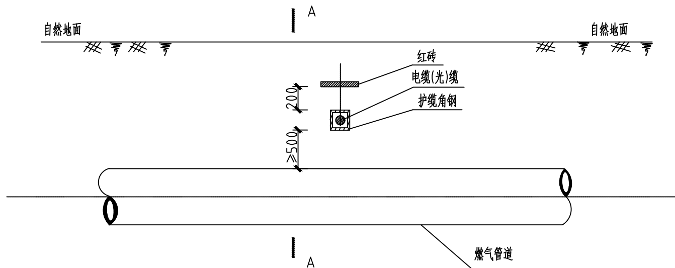
管道穿越电(光)缆断面图
