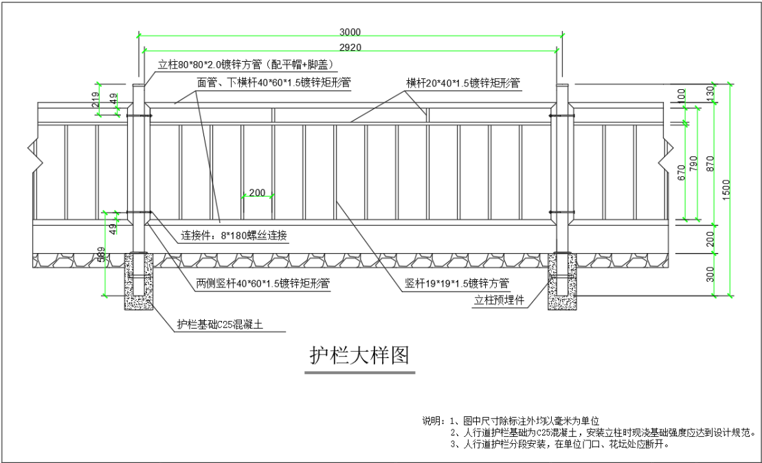
隔离护栏 2 大样图：
