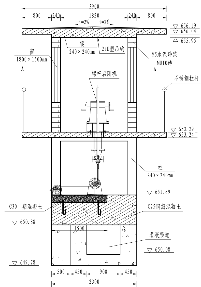
启闭机室剖面图 1:50
