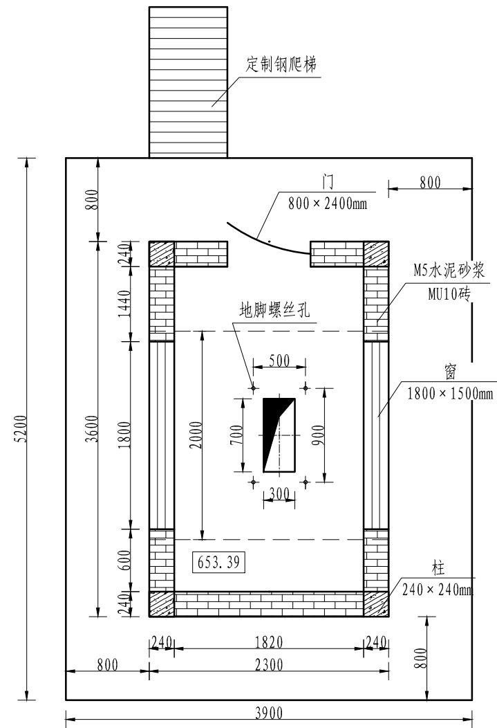
A-A剖面图 1:50
