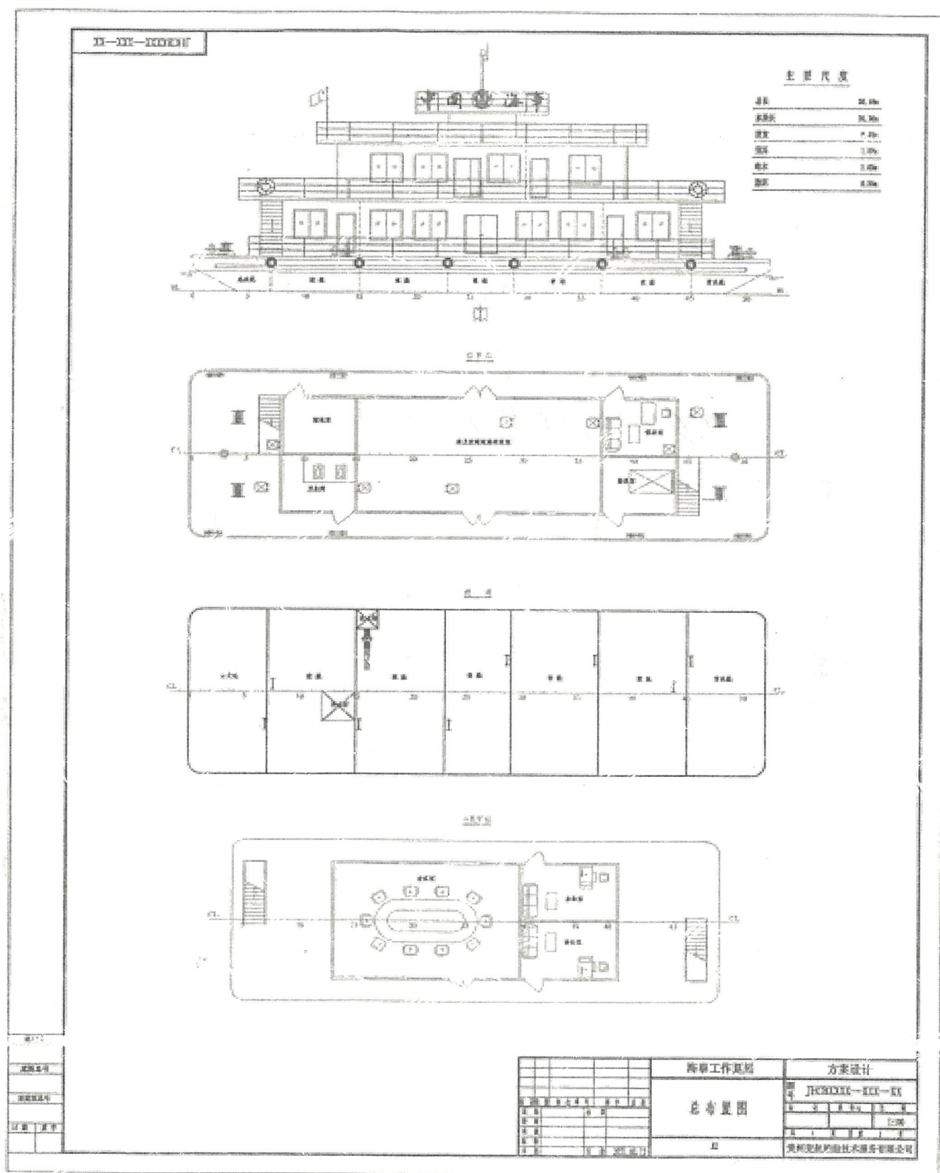
附件一：海事监管趸船总布置图
