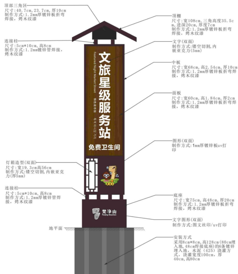
施工图
