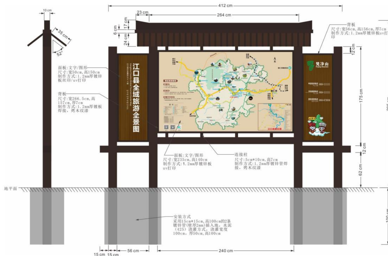
施工图
