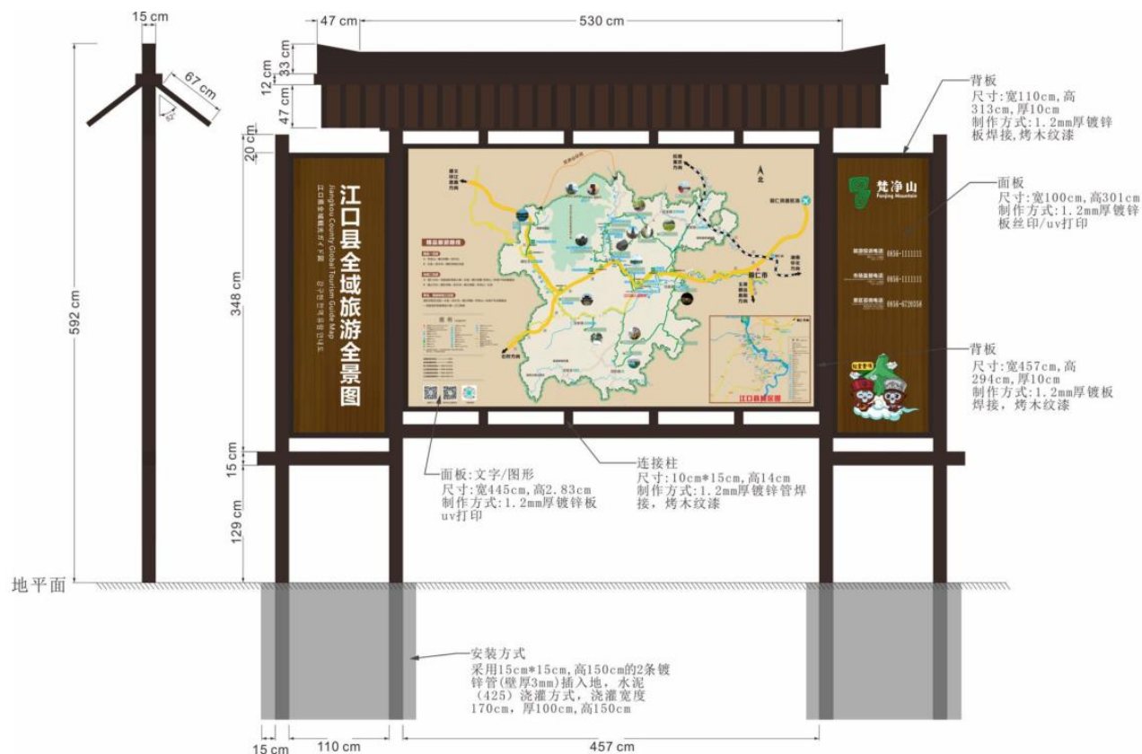
施工图
