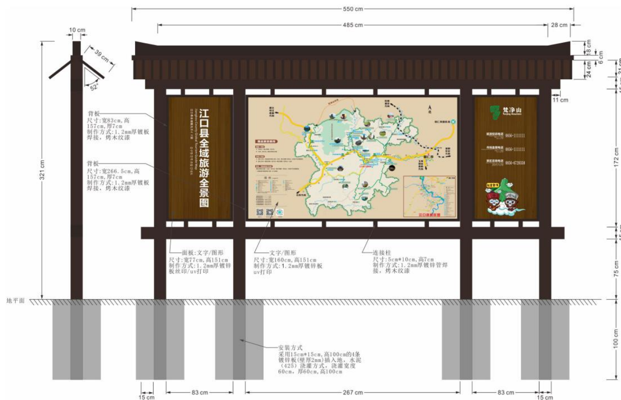
施工图
