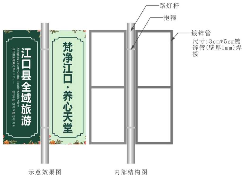
施工图
