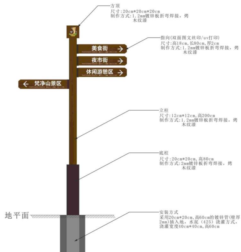
施工图
