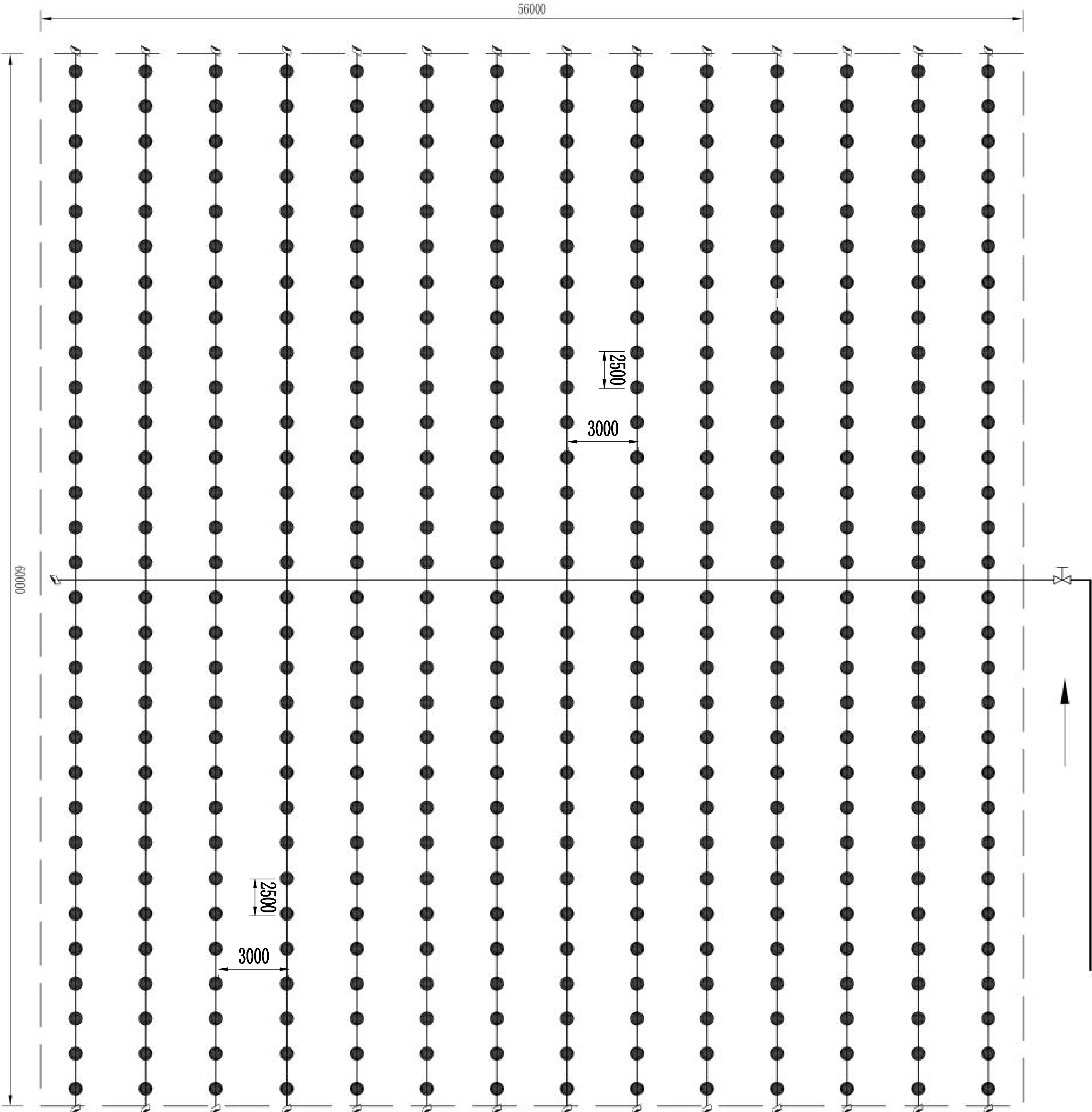
单个灌水单元喷头典型布置图二 1:250
