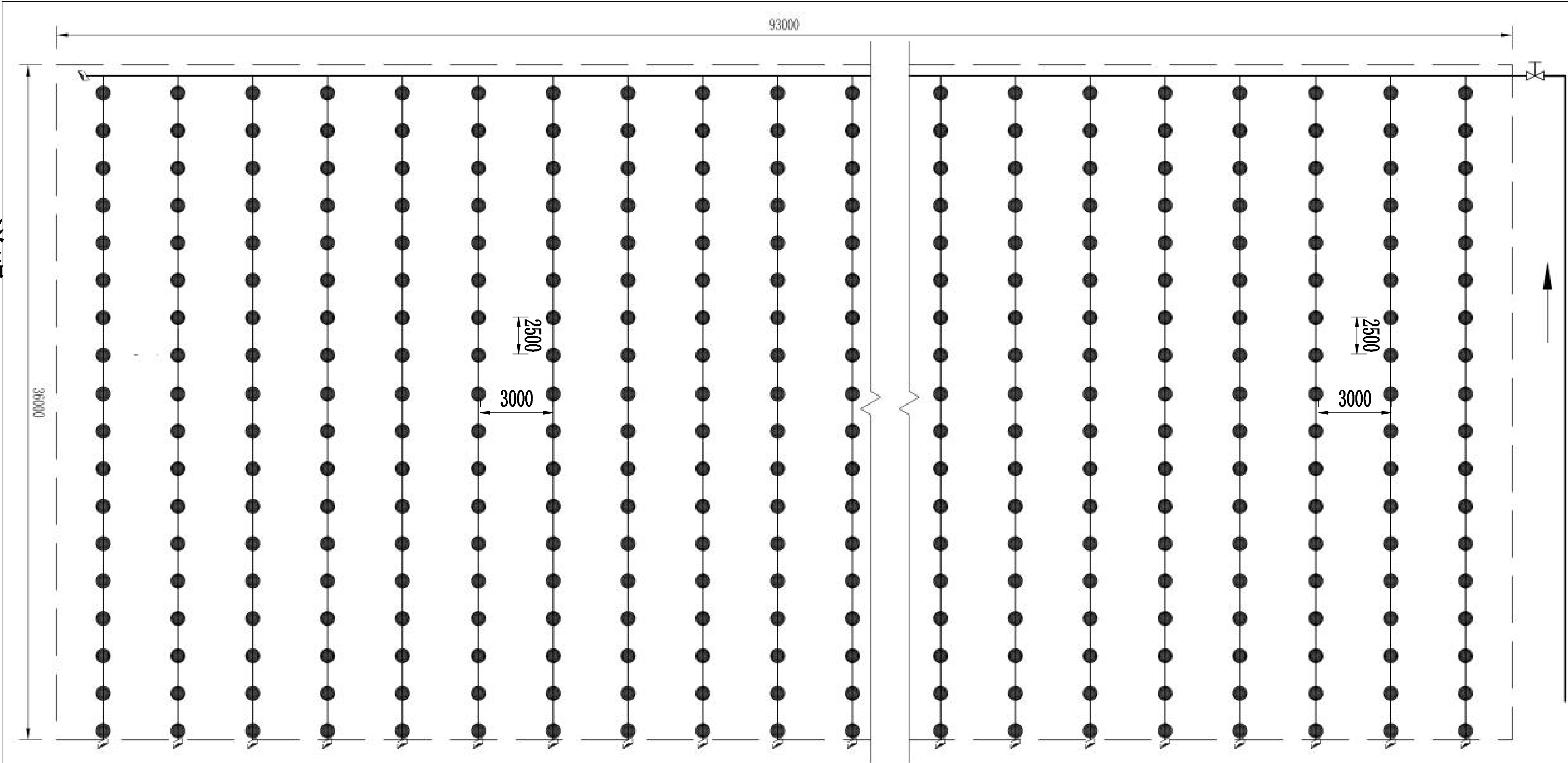
单个灌水单元喷头典型布置图一 1:250
