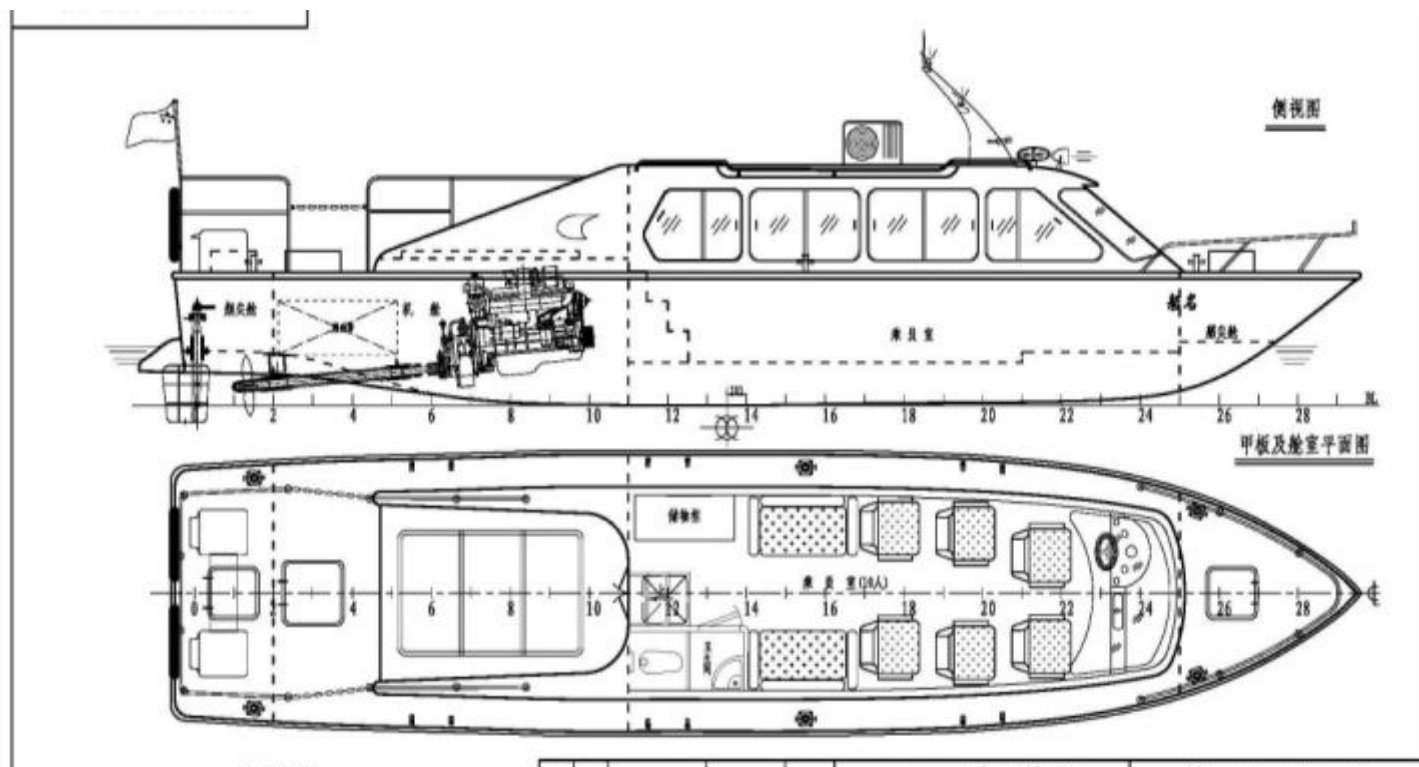
(2) 参考总布置图
