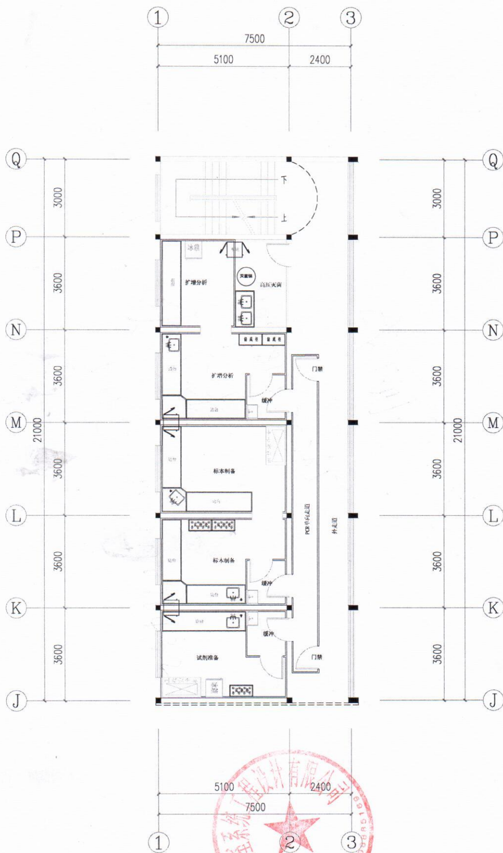
铜仁县思南中医院PCR实验室 1:100
