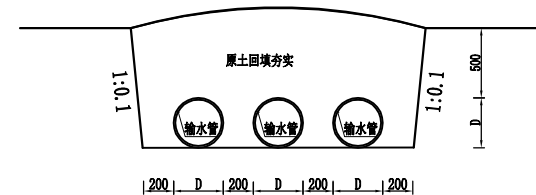
输水管安装横剖面图3 1:50
