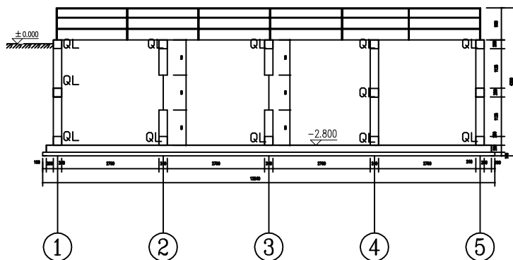
1-1 剖面图
