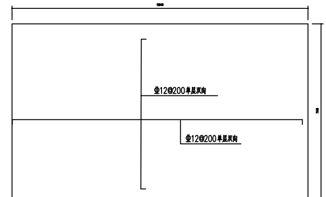
沼液过滤池 池底配筋图
