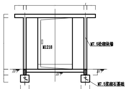
泵房前视图
