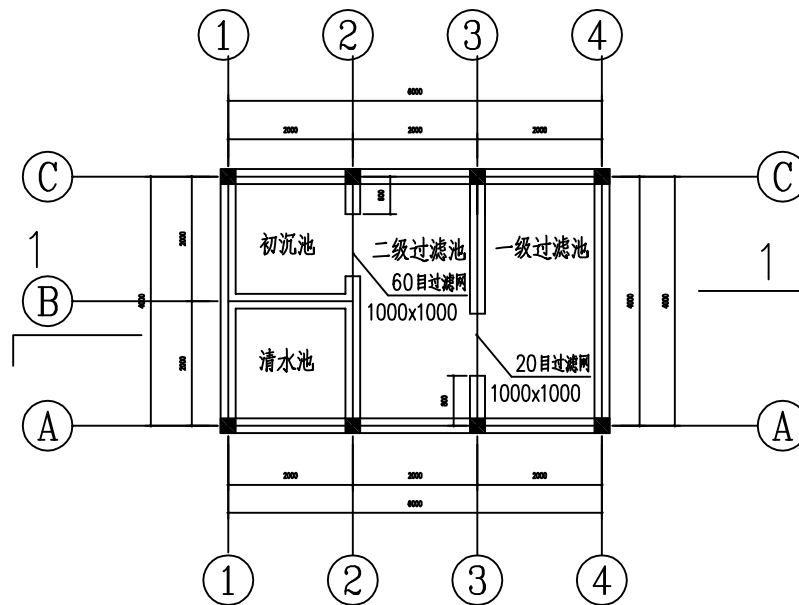
50立方米沼液过滤池平面图
