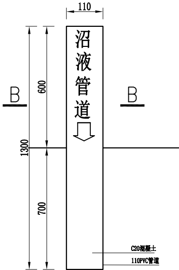
标志桩设计图 1:10
