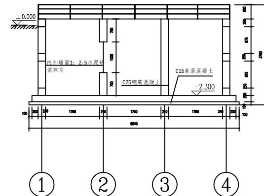
1-1 剖面图
