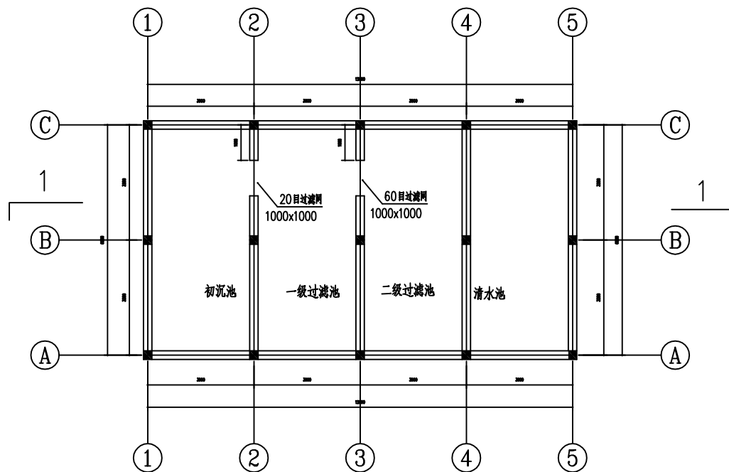
200m³沼液过滤池平面图
