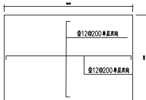
沼液过滤池池底配筋图
