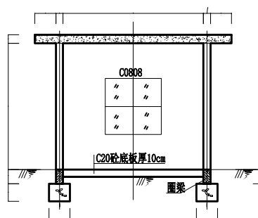
泵房后视图
