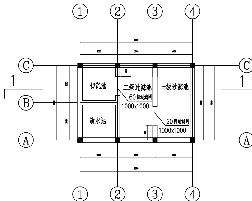
50立方米沼液过滤池平面图
