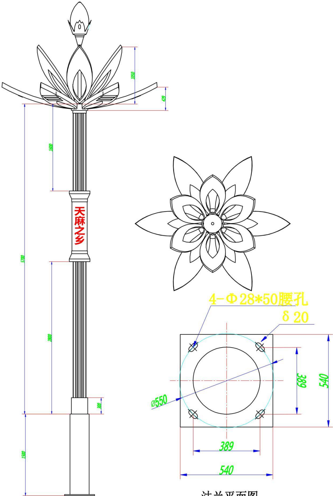
法兰平面图
