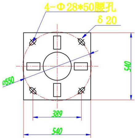
法兰平面图
